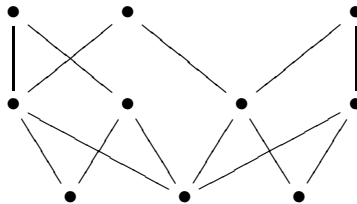
Fig. 4: W \setminus \{x\}
